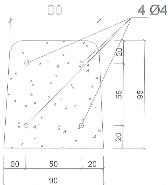
ESTEIO ET9-1
